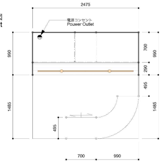
●平面図 Layout
